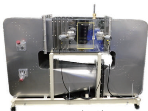
風洞部（本体）
